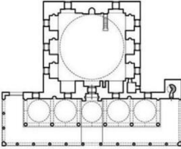
Halep Adiliye Camii 1556 Mimar Sinan
